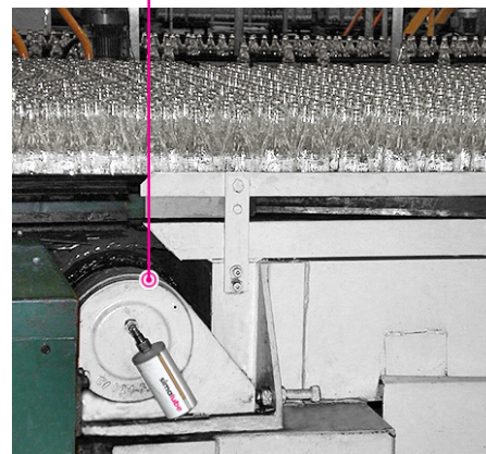
Smering van de aandrijving van een transportband.
