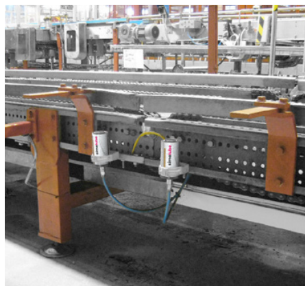
Twee simalube smeerpatronen verlengd met slangen smeren een transportketting in een brouwerij.
