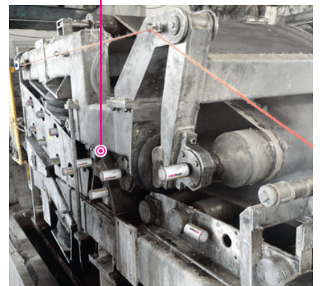
Plusieurs simalube 125 ml lubrifient automatiquement et avec précision les paliers d'une machine à papier.
